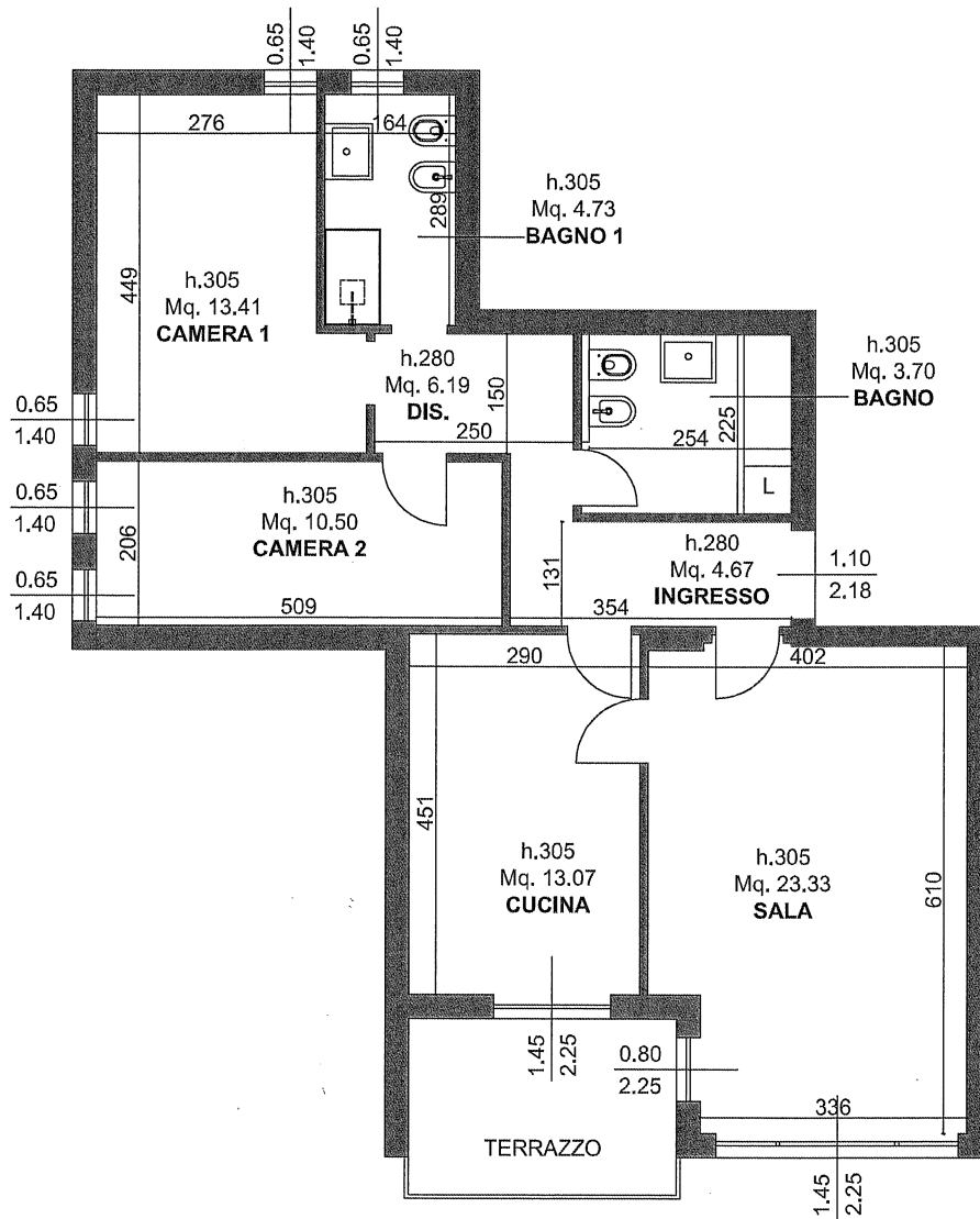
PIANTA PIANO PRIMO STATO FINALE
